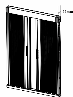
ROYAL 22 PLUS ΔΙΦΥΛΛΗ ΚΕΝΤΡΙΚΗ
